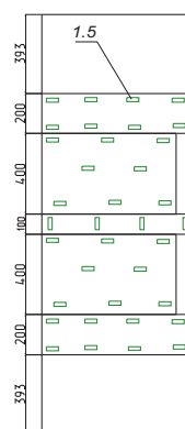
Схема наклейки стекла и зеркал
