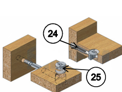
Эксцентриковая стяжка
