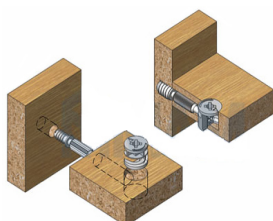
Стяжка эксцентриковая
