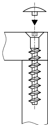
Евровит
