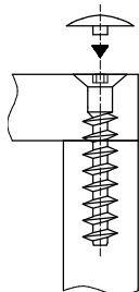
Евровинт 7 x 50
