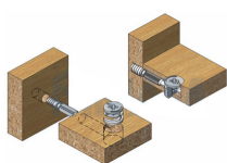
Эксцентриковая стяжка
