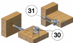
Эксцентриковая стяжка
