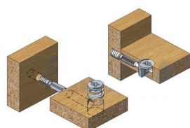
Эксцентриковая стяжка
