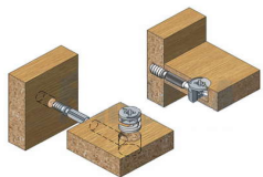
Эксцентриковая стяжка
