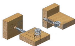
Эксцентриковая стяжка
